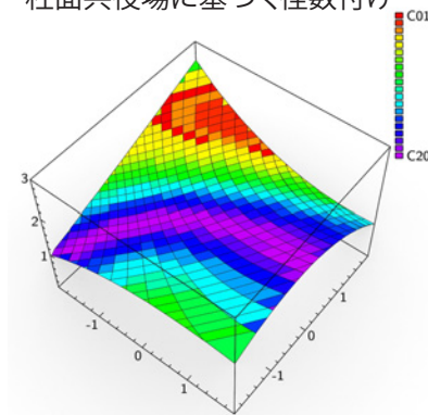
パネリング後のCylindricalStripの連続性
